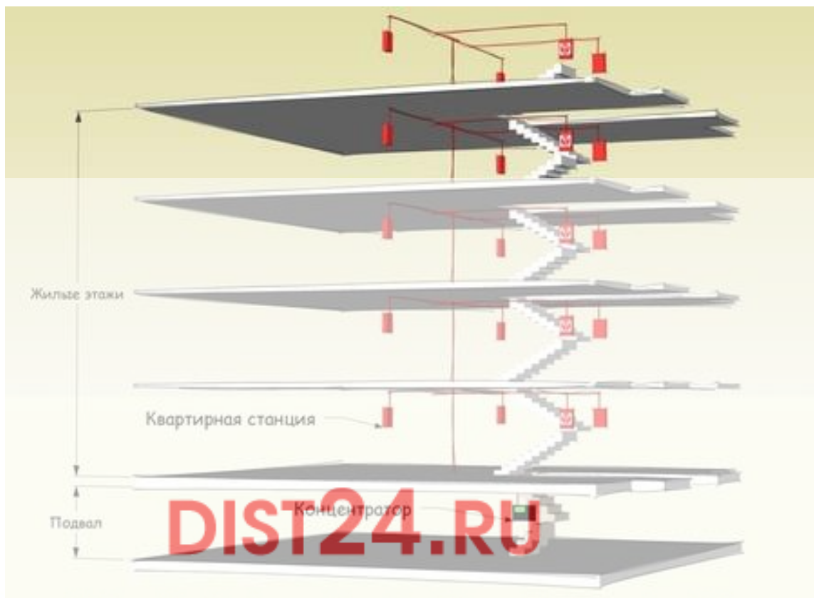
8 Рисунок 5 – Структура сбора данных по сети стандарта M-Bus 8 (800) 100-62-72
